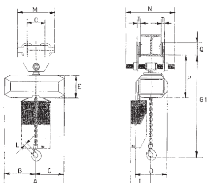
Tipo a Traslazione a Spinta
