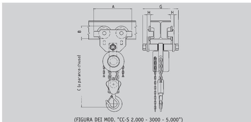
(FIGURA DEI MOD. "CC-S 2.000 - 3000 - 5.000")
