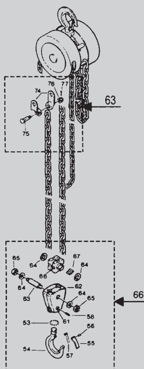
Paranco a 2 tiri di catena
