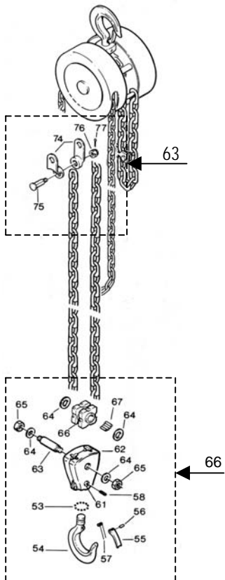
Paranco a 2 tiri di catena
