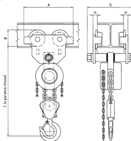
(Figura del Mod. "CC-S 2.000 al Mod. "CC-S 5.000")
